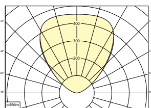
MI04023040 40w 4000k 7.200lm ηLB 93,4%
